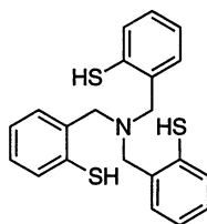
tris(2-mercaptobenzyl)amine (S 3 N)
