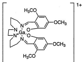
Ga((4,6-MeO 2 sal) 2 BAPEN)
